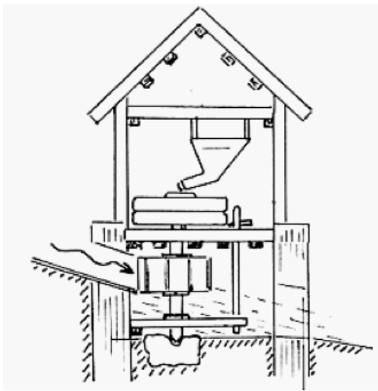
Skvatmølle (tegning)
